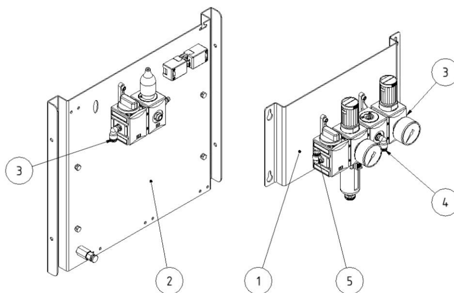
Fig. 13: trykkluftenhet (Outdoor-versjon)
