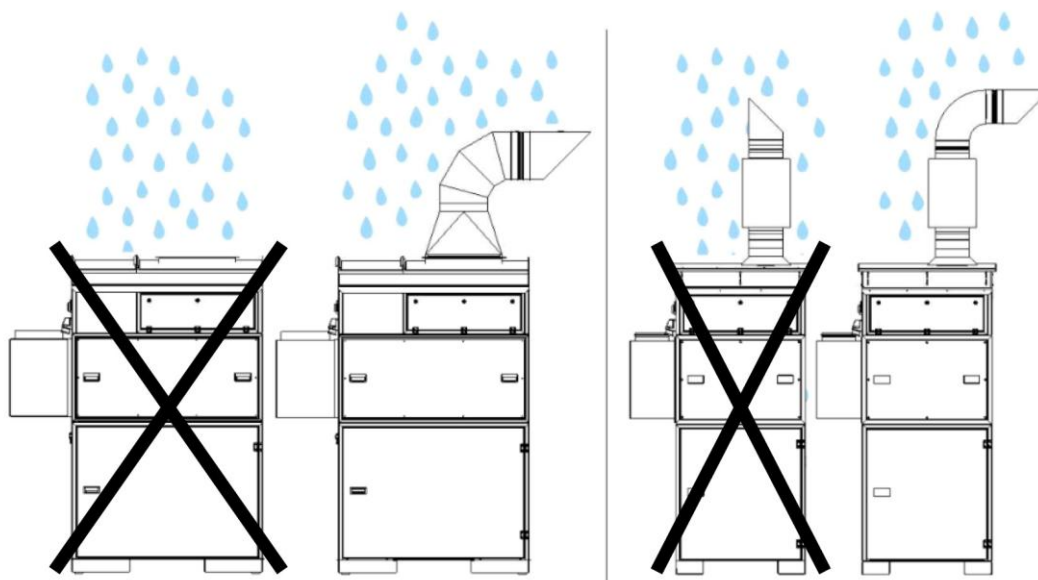
Fig. 9: Outdoor-versjon
