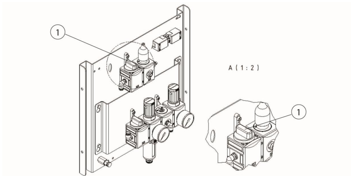
Fig. 37: trykkluftventil støvsamlebeholder
