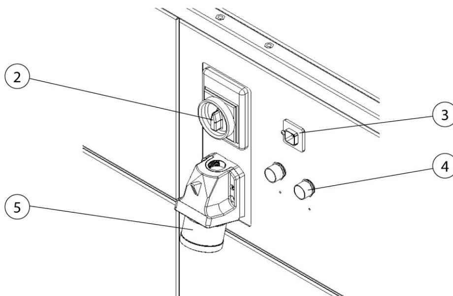
Fig. 7: tilkoblingspaneler
