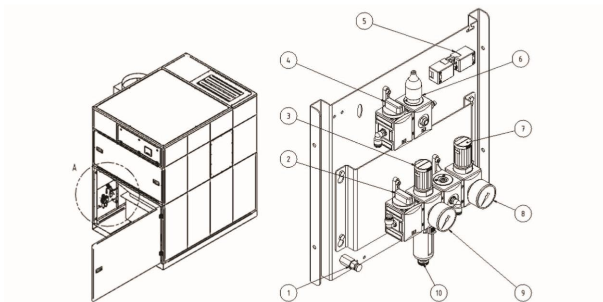
Fig. 12: trykkluftenhet
