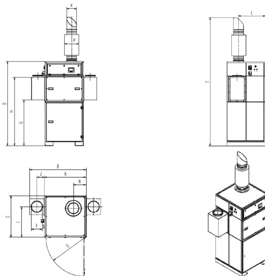
Fig. 58: måleblad 3420
