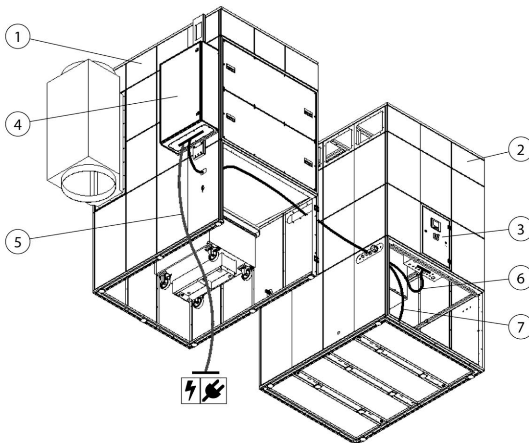
Fig. 15: Eksempel: Kabellegging sugееffektregulering
