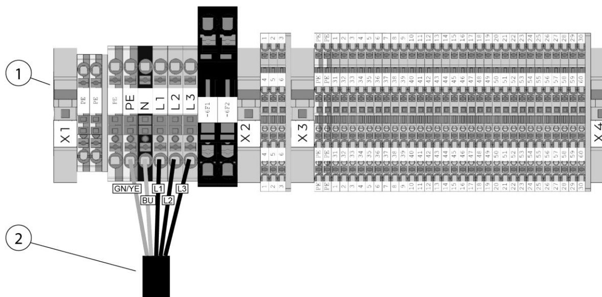
Fig. 14: tilkoblingsrekkeklekke koblingsskap produkt
